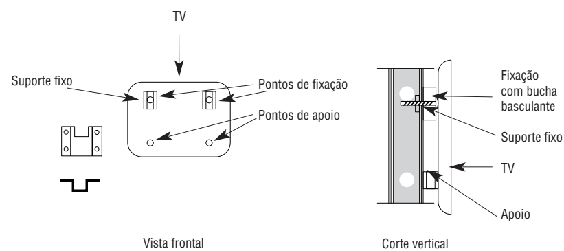
TV rente à parede com suporte fixo
